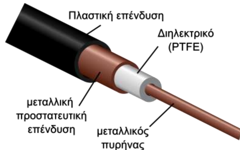
Σχηματική απεικόνιση τομής ηλεκτρικού καλωδίου
