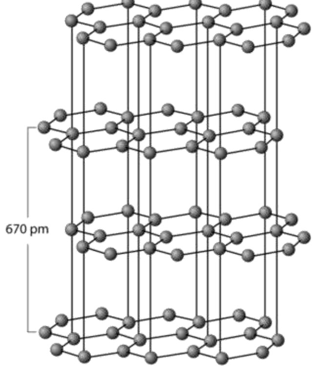
Δομή Γραφίτη
