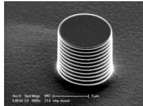
Εικόνα SEM από ion etching (Si pillar)
