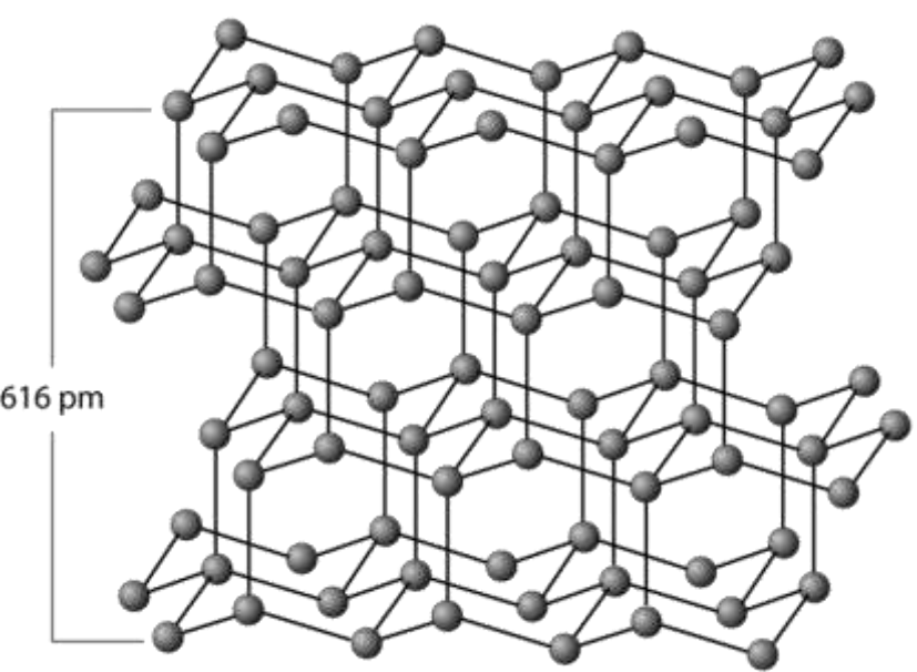
Δομή Διαμαντιού
