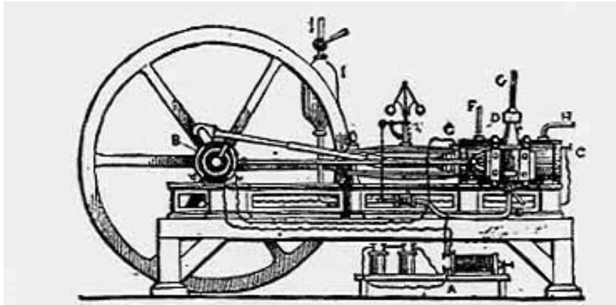
Μηχανή εσωτερικής καύσης Lenoir, 1860
