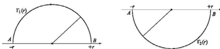
Σχ. 4: Κλειστοί δρόμοι ολοκλήρωσης που χρησιμοποιούνται στον υπολογισμό πραγματικών ολοκληρωμάτων με άπειρα όρια.
