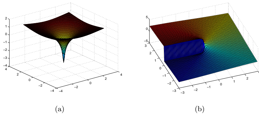
Σχήμα 1.4: Γραφική παράσταση του πραγματικού και του φανταστικού μέρους της λογαριθμικής συνάρτησης.
