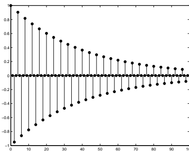
Σχήμα 6.7: Η κρουστική απόκριση ενός συστήματος δεύτερης τάξης με δύο μιγαδικές ρίζες.
